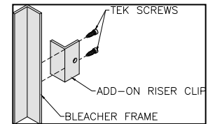
Riser Bracket
