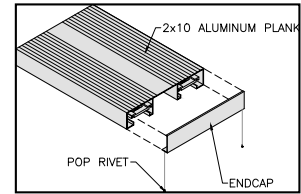
End Cap
